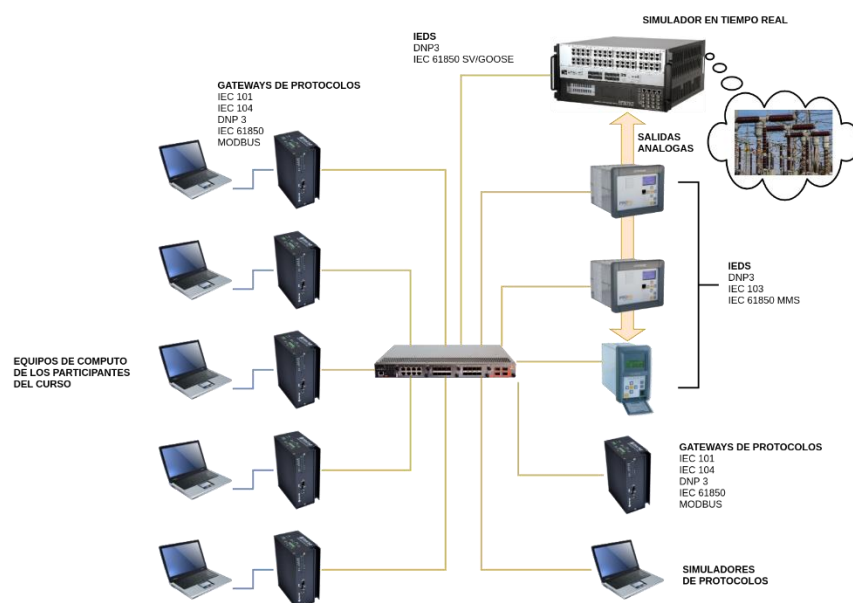
Figura 1. Arquitectura a implementar para la sesión práctica en DNP3, IEC101/104
